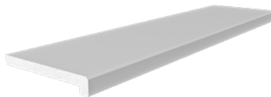
Cod: SOGLIAZERO Copri soglia in EPS sagomata e resinata Dimensioni: mm 1500 x 450 x 60/30 mm 2000 x 450 x 60/30 mm 1500 x 350 x 60/30 mm 2000 x 350 x 60/30
